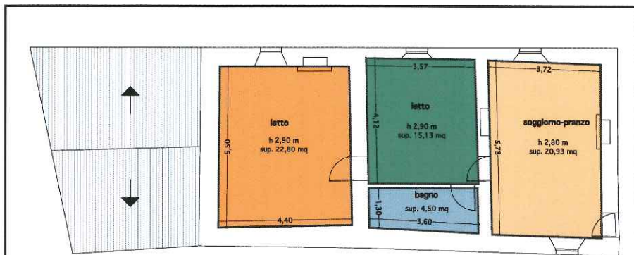
pianta quotata
